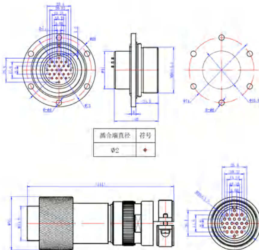
图 12 DTU26 芯航插 (电流输入与控制信号) 插座、插头尺寸
